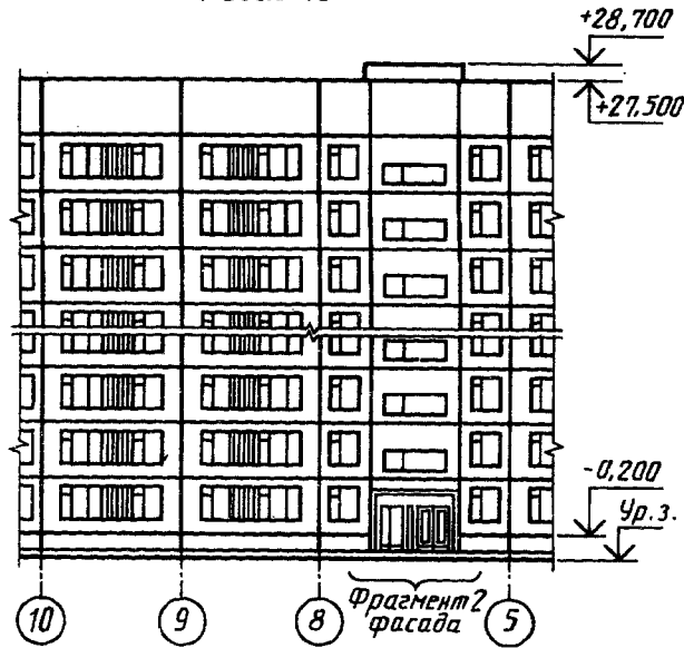
Фасад 10-5
