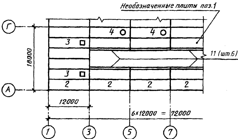
Схема расположения плит покрытия
