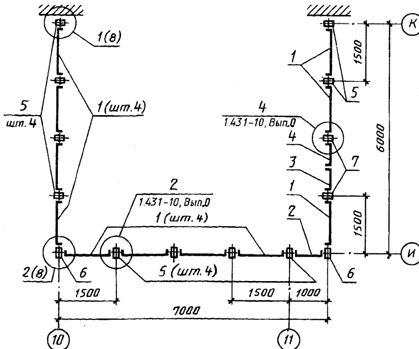
Пример выполнения схемы расположения элементов, сборных перегородок
